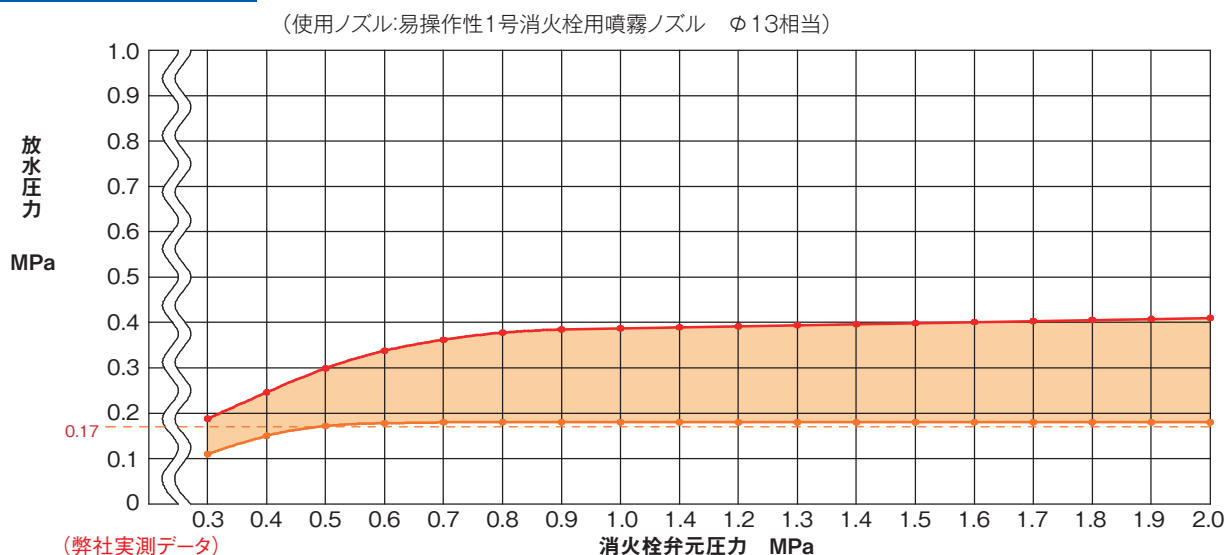
易操作性1号消火栓(バセットII)性能表
