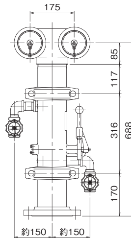
1.6MPa仕様
