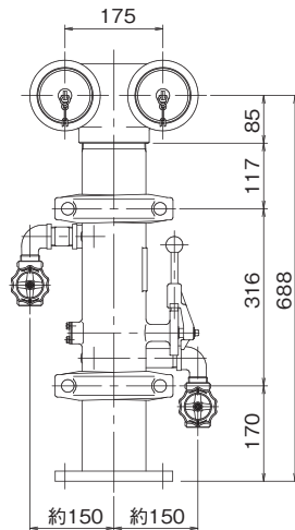
1.4MPa仕様
