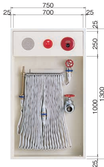
B123 横二段単独型
