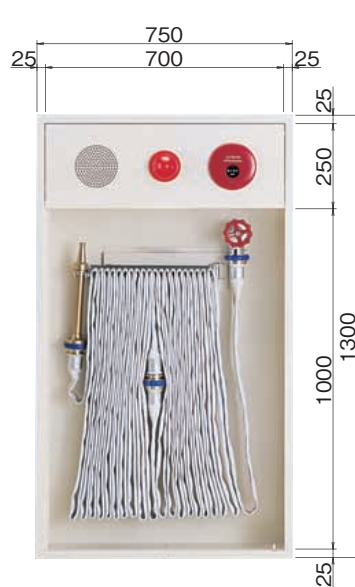
B130 二段単独型 Wタイプ
