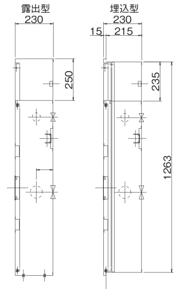
B130格納状態 ポンプ起動押釦付の場合 Wタイプ
