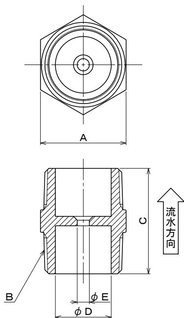
寸 法
