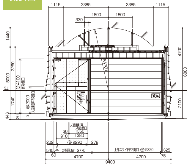
連絡坑 側姿図
