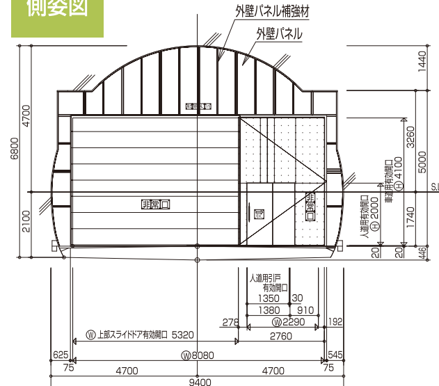
車道 側姿図
