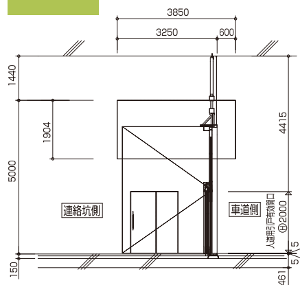
A-A 断面図
