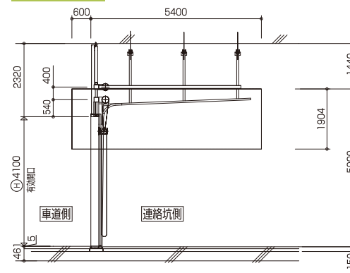
B-B 断面図
