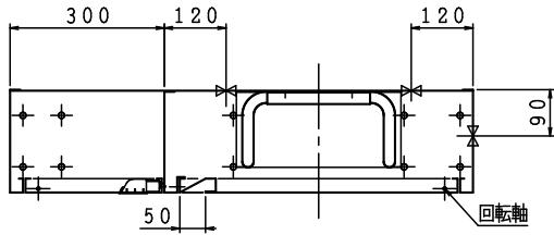
露出形 HB-4BS
