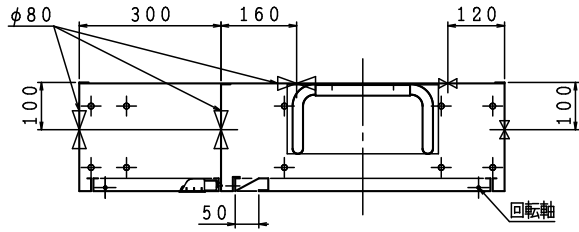
露出形 HB-4BS
