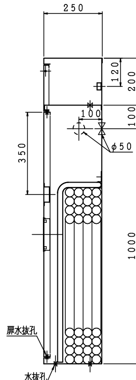
露出型
