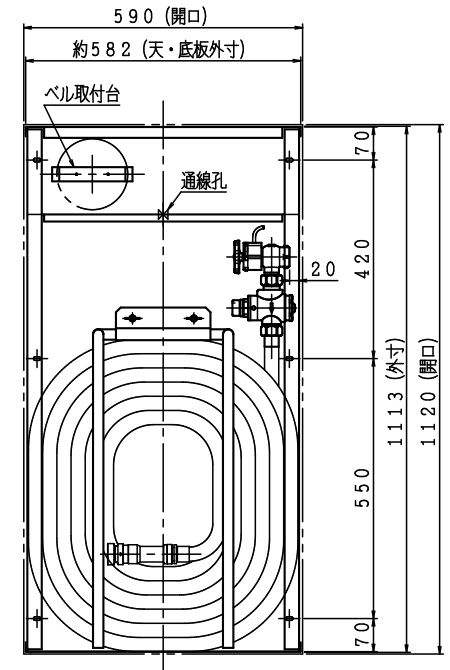
注) 横配管時、側板と消火栓の面間は図中記入寸法をお守り下さい。
