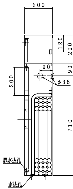
露出型
