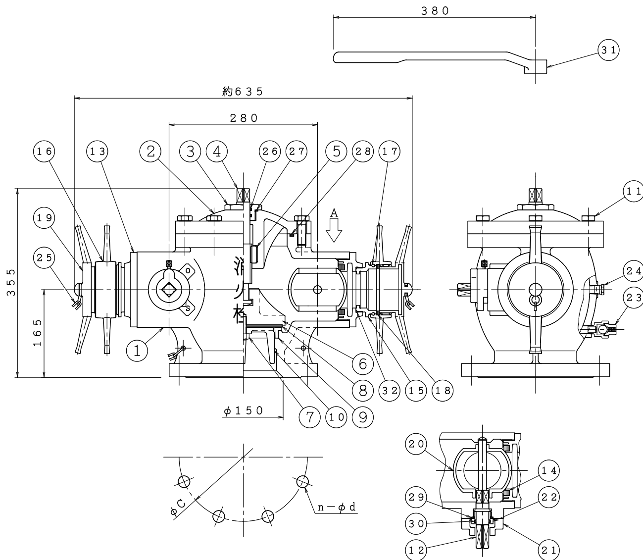
矢視A 断面図
