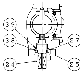
矢視A 断面図
