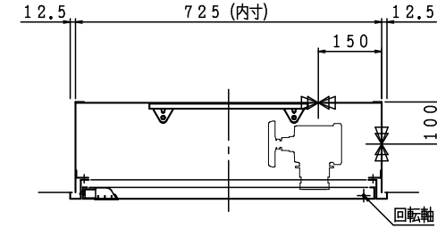
埋込型 注) 本体前面は壁仕上面より前に出さないで下さい。
