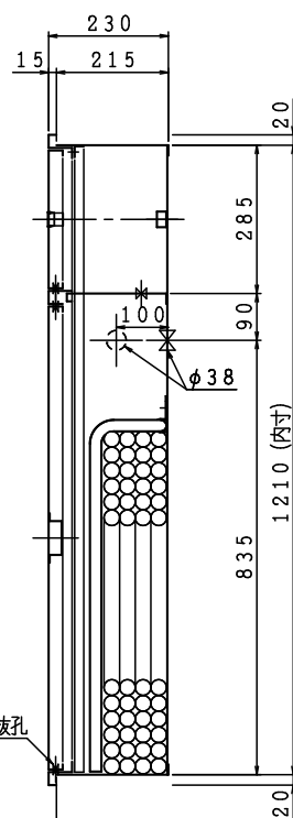
埋込形 HB-4AS
