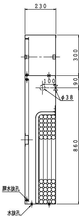
露出形 HB-4BS
