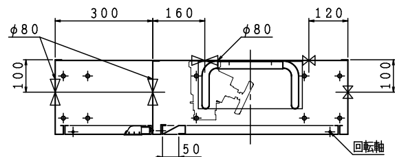
露出形 HB-4BS
