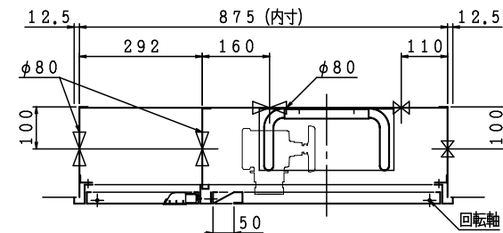
埋込形 注) 本体前面は壁仕上面より前に出さないで下さい。 HB-4AS
