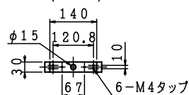
端子・ベル取付台 (H: 20)
