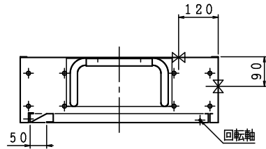
露出形 HB-4B
