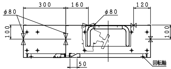
露出形 HB-4BS
