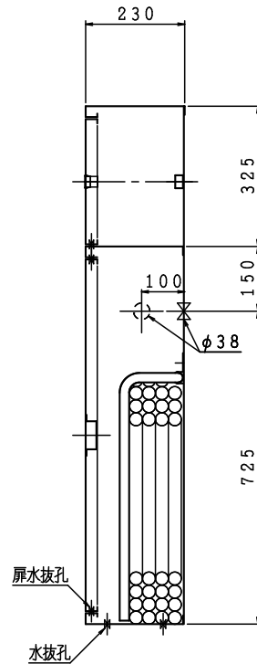
露出形 HB-4BS
