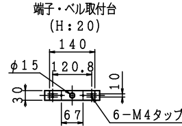
埋込形 HB-4AS
