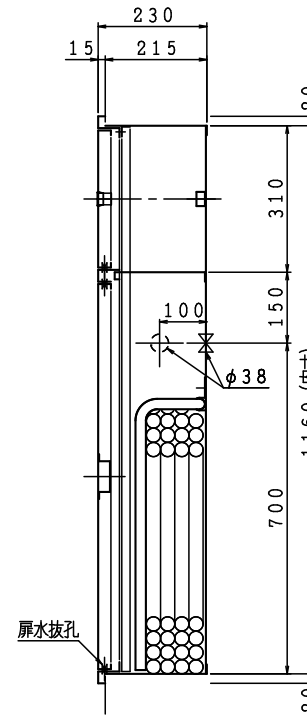
埋込形 HB-4AS
