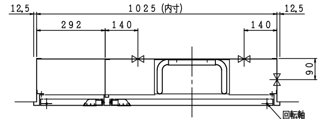
埋込型
