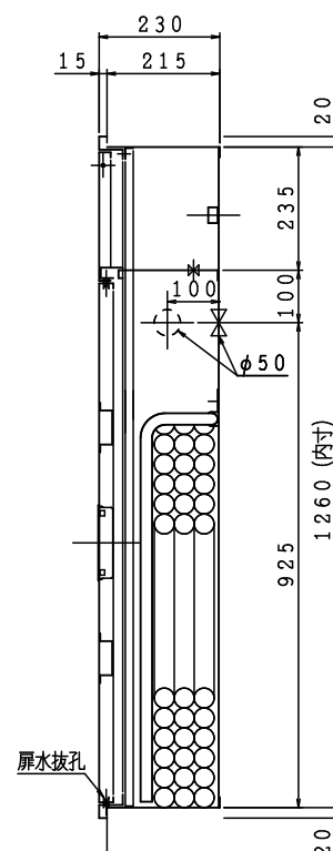
埋込型
