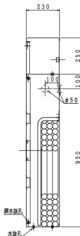
露出型
