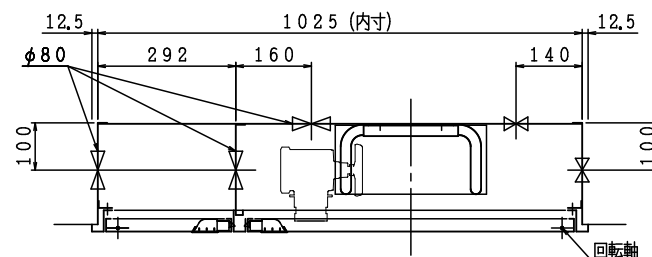
埋込型
