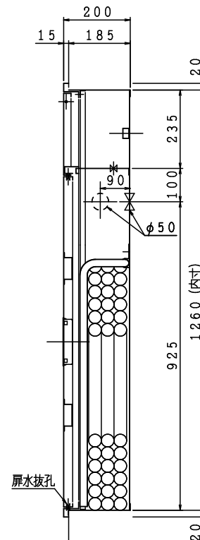
埋込型
