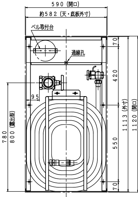
注）横配管時、側板と放水口の面間は図中記入寸法をお守り下さい。
