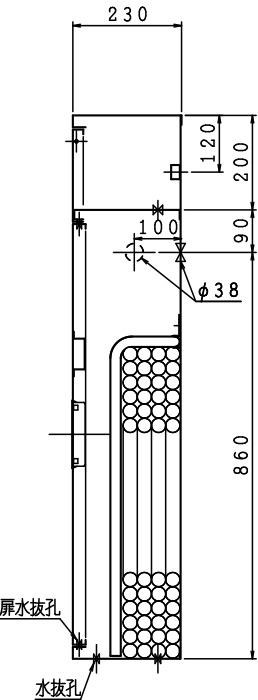
露出型
