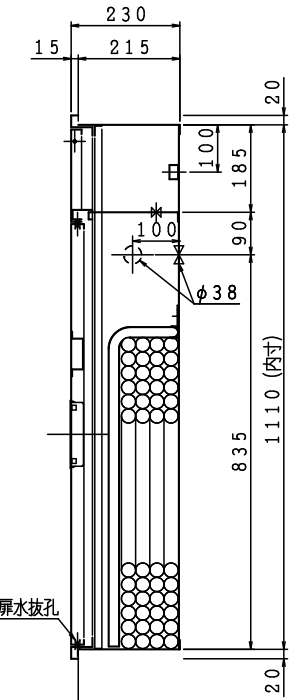
埋込型
