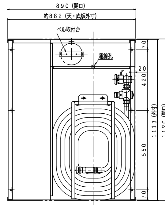
注) 横配管時、側板と消火栓及び放水口の面間は図中記入寸法をお守り下さい。
