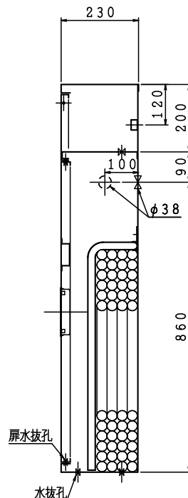
露出型
