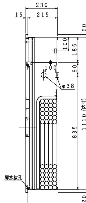
埋込型
