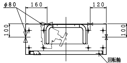
露出型
