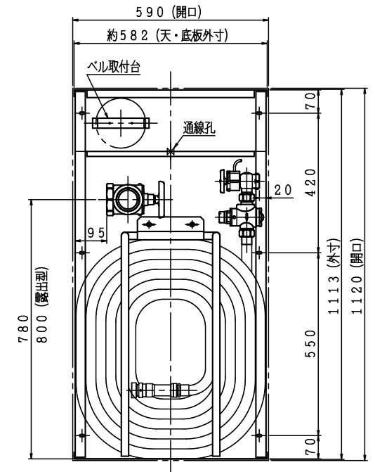
注) 横配管時、側板と消火栓及び放水口の面間は図中記入寸法をお守り下さい。
